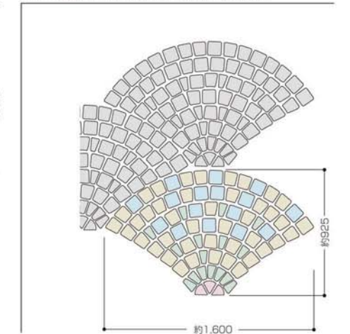
ウロコ張り半径約925mm 0.85㎡の使用材料
