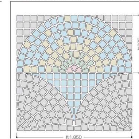
半円張り半径約1,850mm×925mm 1.71㎡の使用材料
