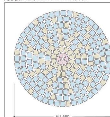
円形張り半径約925mm 2.68㎡の使用材料
