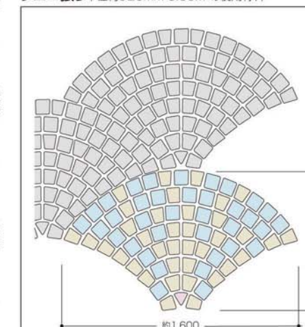
ウロコ張り半径約925mm 0.85㎡の使用材料
